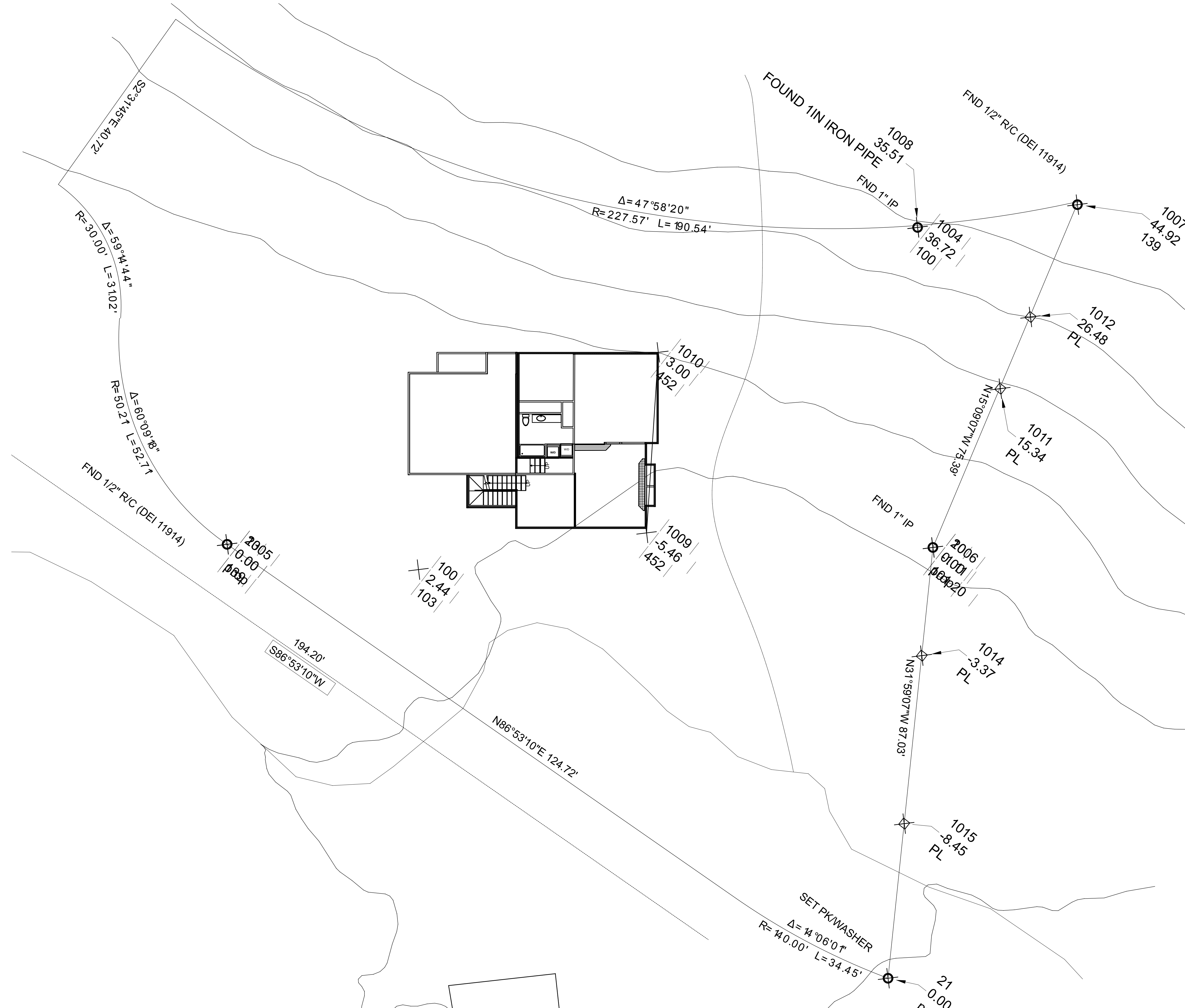
1 Boundary Survey A2 SCALE: 1" = 10'
